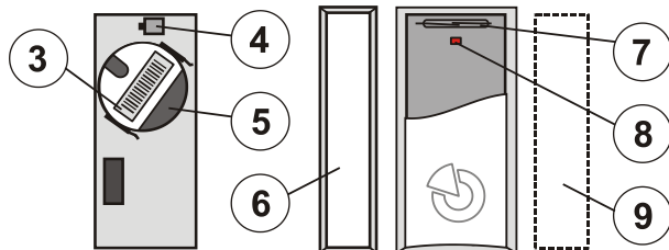
Rysunek: 3 – kod produkcji; 4 – styk anty-sabotażowy; 5 – bateria; 6 – magnes; 7 – sensor magnetyczny; 8 – czerwony wskaźnik aktywacji czujki; 9 – alternatywne położenie magnesu
